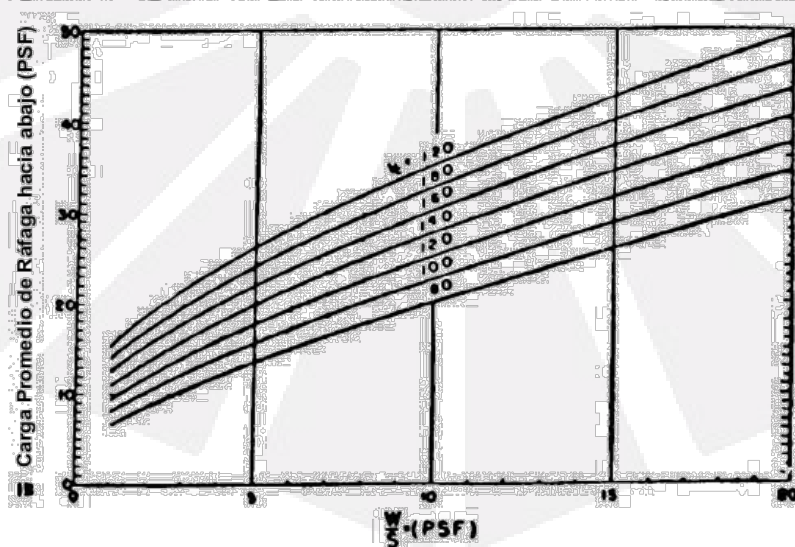
Figura 3. Carga de Ráfaga hacia abajo en superficie del Empenaje Vertical
