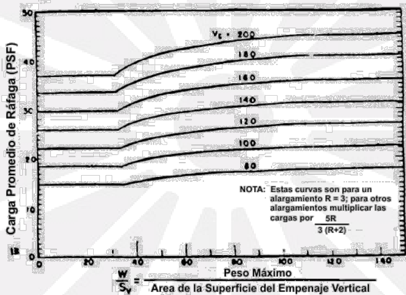
Figura 5. Carga de Ráfaga en Superficie del Empenaje Vertical
