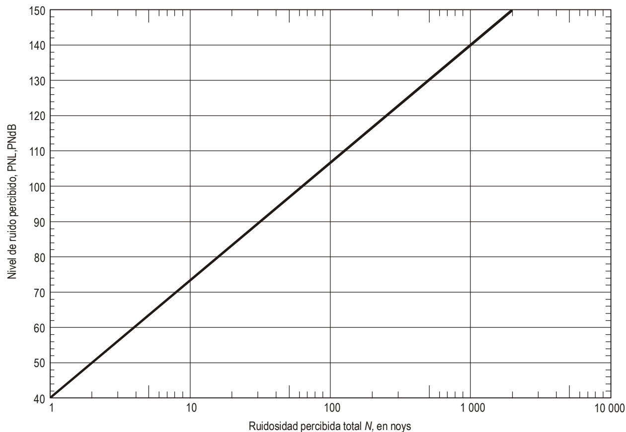
Figura A1-1. Nivel de ruido percibido en función de la ruidosidad percibida total
