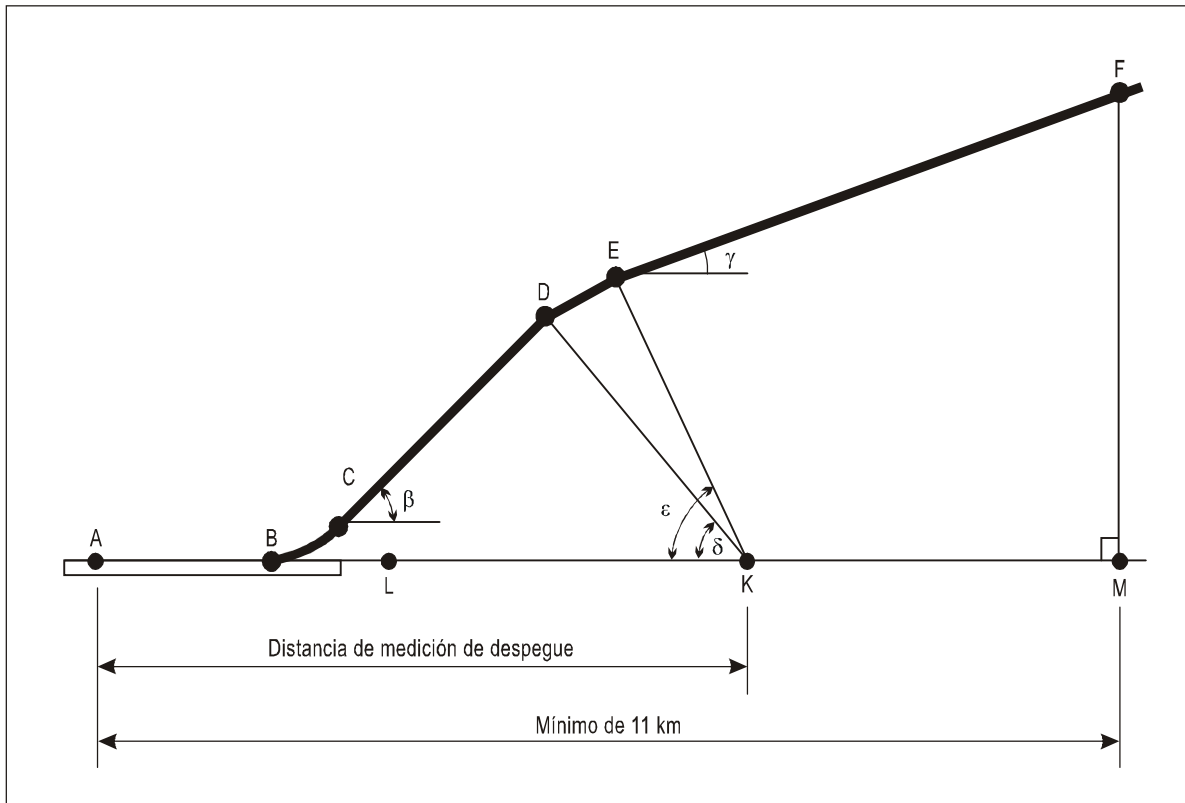
Figura A1-4. Perfil de despegue medido
