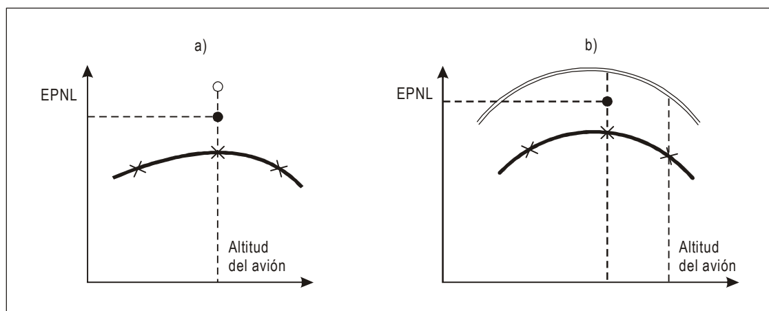
Figura A2-13. Corrección de asimetría lateral
