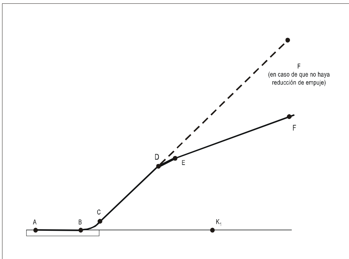
Figura A2-5. Características del perfil de sobrevuelo de referencia para aviones
