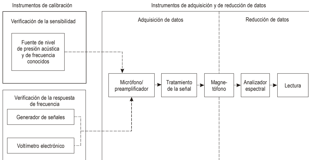
Figura C-1. Sistemas de medición del ruido
