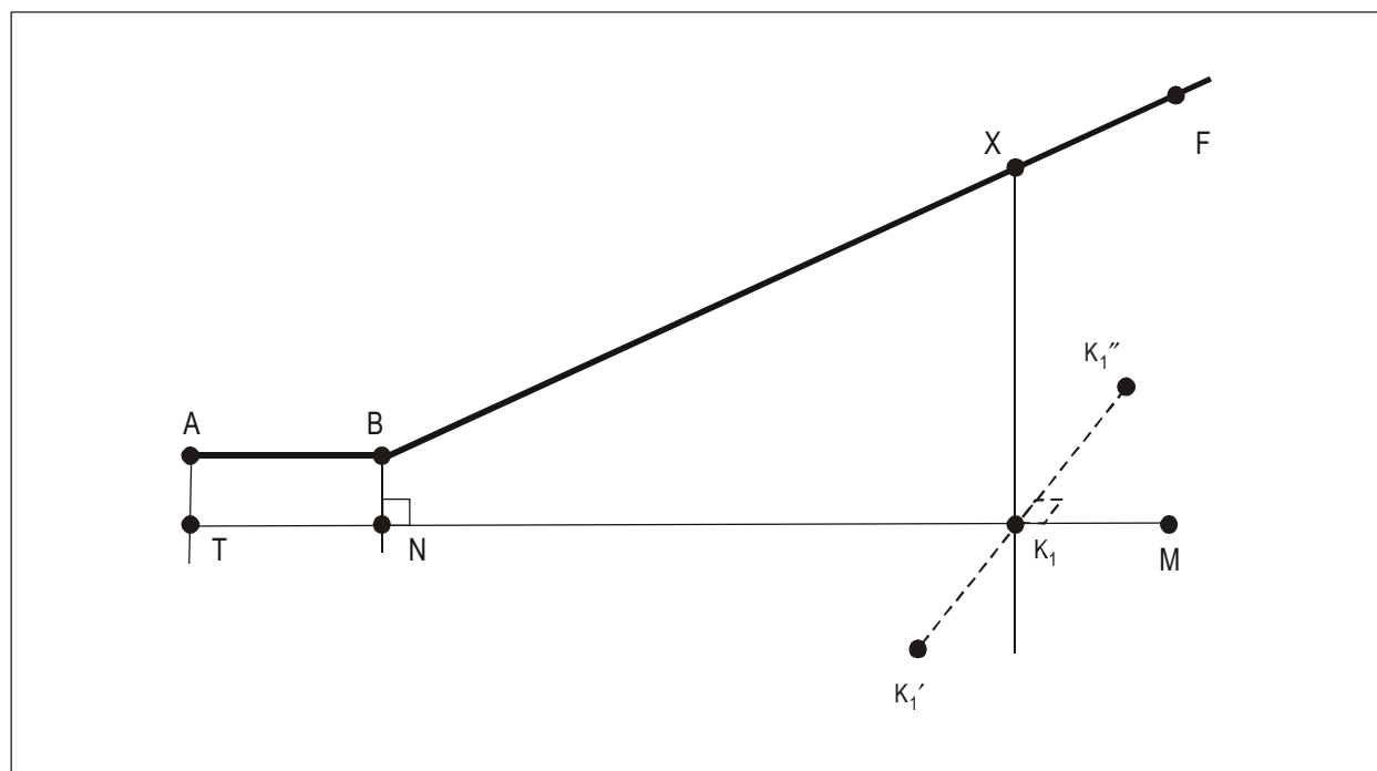
Figura A2-7. Características del perfil de despegue de referencia para helicópteros
