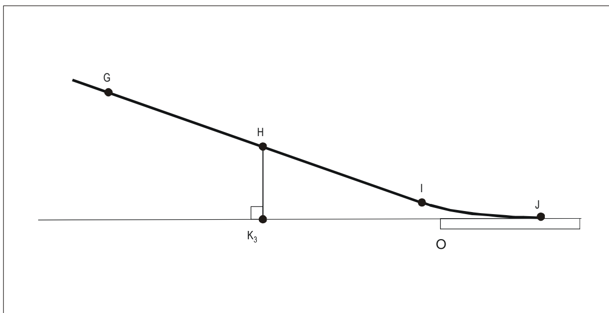
Figura A2-6. Características del perfil de aproximación de referencia para aviones
