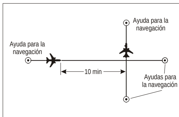
Figura 5-15. Separación de 10 minutos entre aeronaves por derrotas que se cruzan y al mismo nivel [véase 5.4.2.2.1.2 b)]
