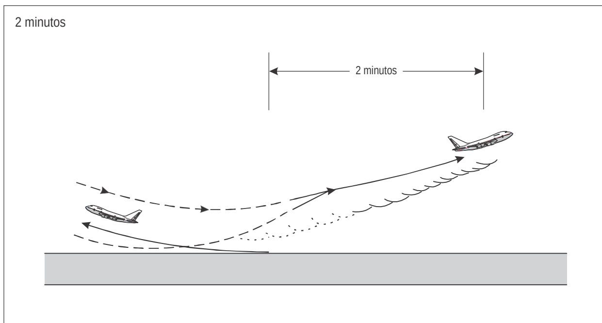
Figura 5-45. Separación de 2 minutos por estela turbulenta para despegue en sentidos opuestos [véase 5.8.5 a)]
