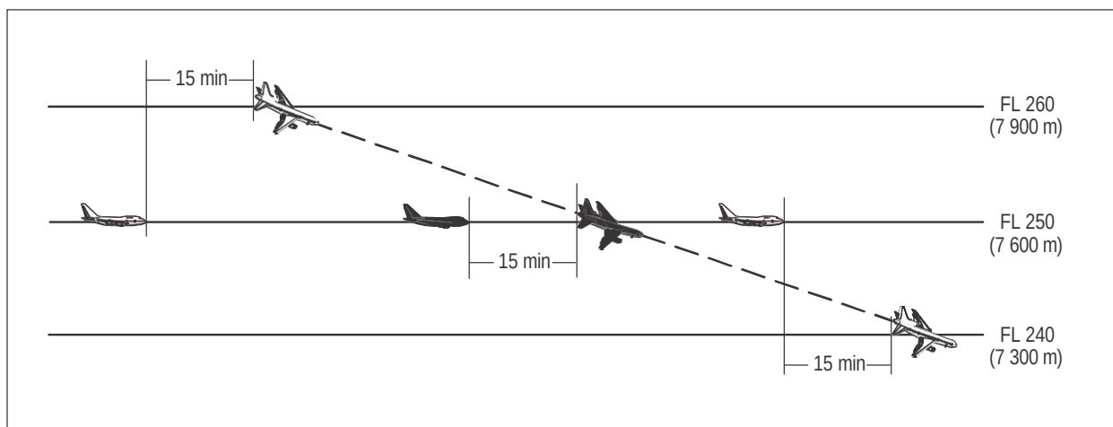
Figura 5-19B. Separación de 15 minutos entre aeronaves que descienden y por derrotas que se cruzan [véase 5.4.2.2.2 a)]
