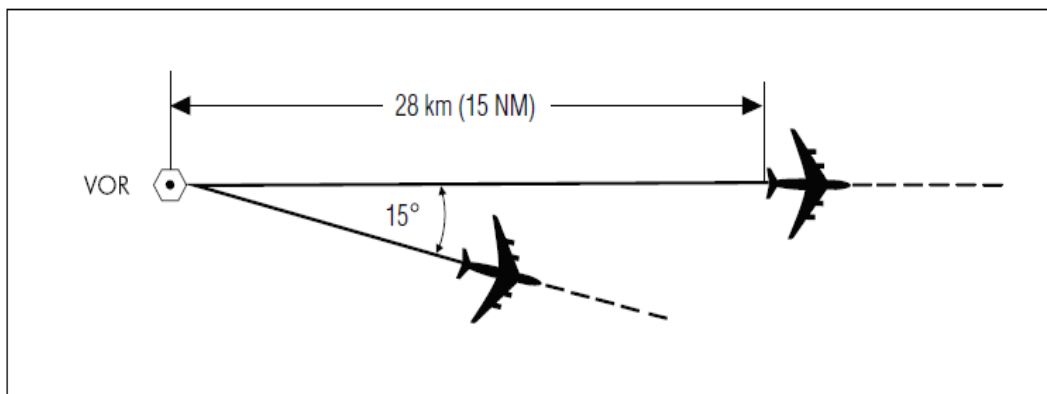
Figura 5-4. Separación utilizando el mismo VOR [véase 5.4.1.2.1.2 a)]
