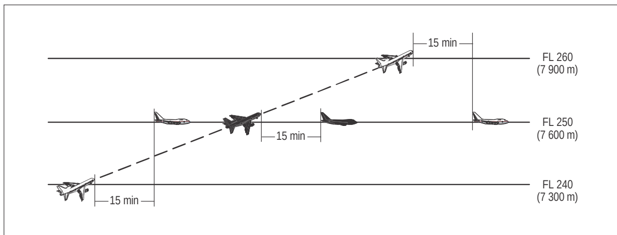
Figura 5-19A. Separación de 15 minutos entre aeronaves que ascienden y por derrotas que se cruzan [véase 5.4.2.2.2 a)]
