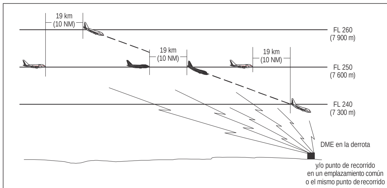
Figura 5-25B. Separación de 19 km (10 NM) basada en DME y/o en GNSS entre aeronaves que descienden y por la misma derrota [véase 5.4.2.3.4.1 c)]
