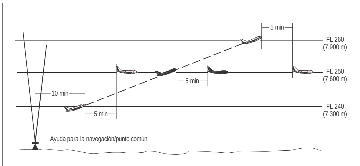
Figura 5-18A. Separación de 5 minutos entre aeronaves que ascienden y por la misma derrota [véase 5.4.2.2.2.1 c) 2)]
