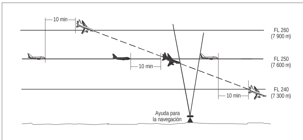
Figura 5-20B. Separación de 10 minutos entre aeronaves que descienden y por derrotas que se cruzan [véase 5.4.2.2.2 b)]
