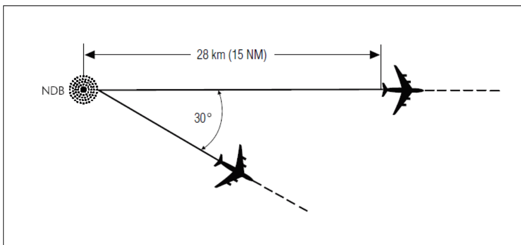
Figura 5-5. Separación utilizando el mismo NDB [véase 5.4.1.2.1.2 b)]
