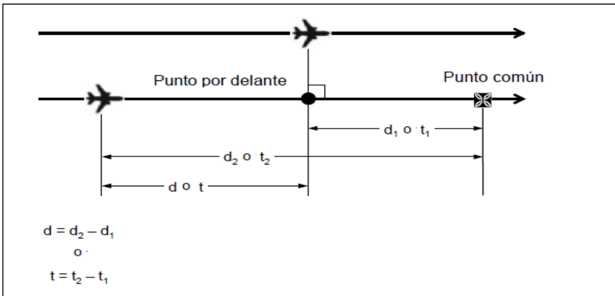
Figura 5-35. Cálculo de la distancia/tiempo longitudinal entre aeronaves — derrota paralela [véase 5.4.2.9.5 c)]
