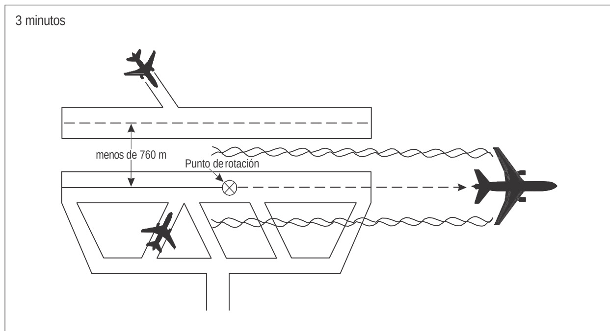
Figura 5-44. Separación de 3 minutos por estela turbulenta para la aeronave que sigue (véase 5.8.3.2)
