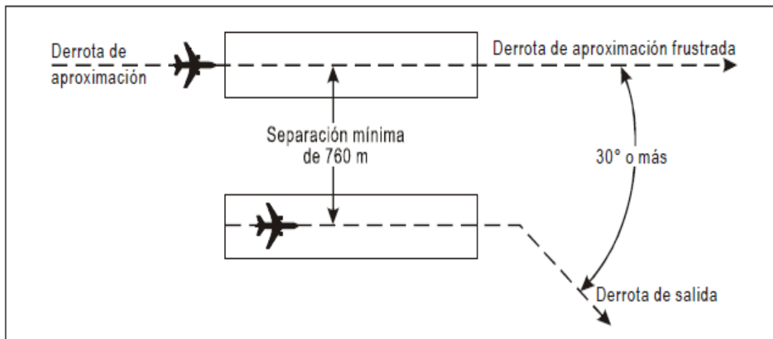
Figura 6-1. Operaciones paralelas segregadas [véase 6.7.3.5.1 b)]
