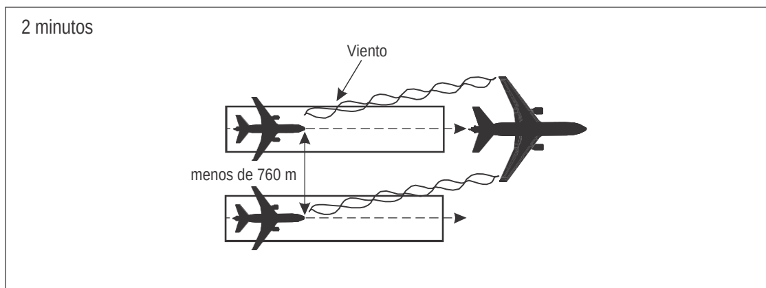
Figura 5-42. Separación de 2 minutos por estela turbulenta para aeronaves que siguen [véase 5.8.3.1 a) y b)]
