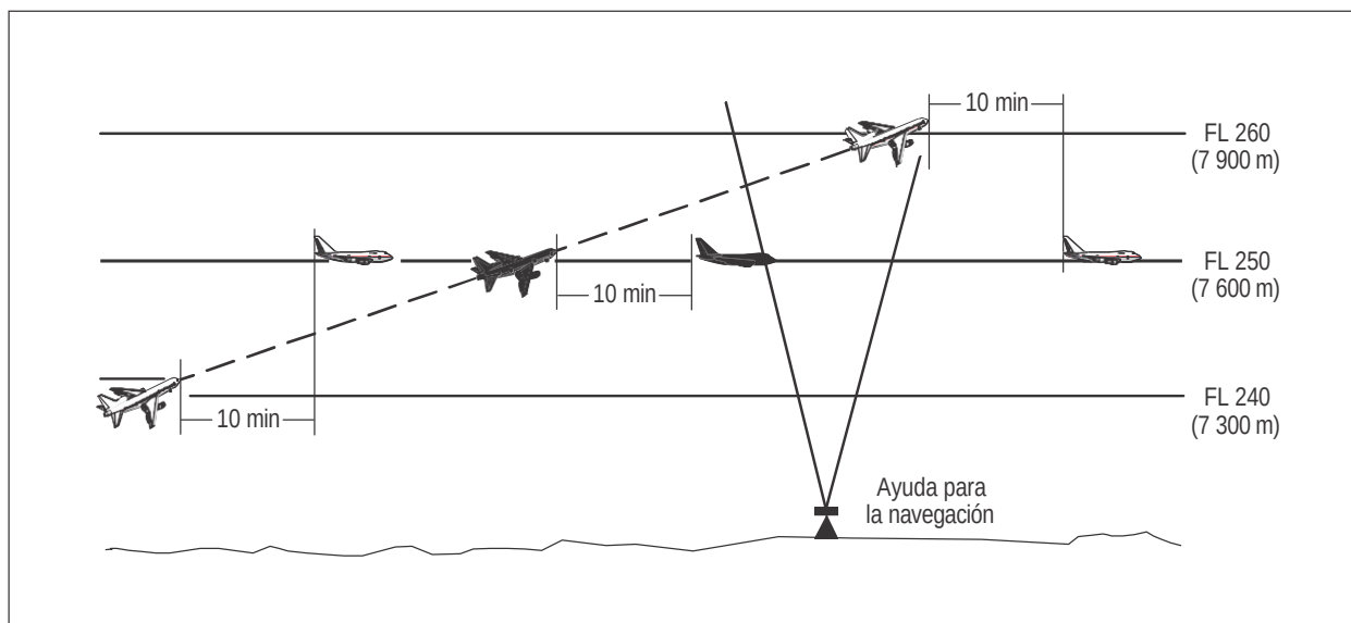
Figura 5-20A. Separación de 10 minutos entre aeronaves que ascienden y por derrotas que se cruzan [véase 5.4.2.2.2 b)]
