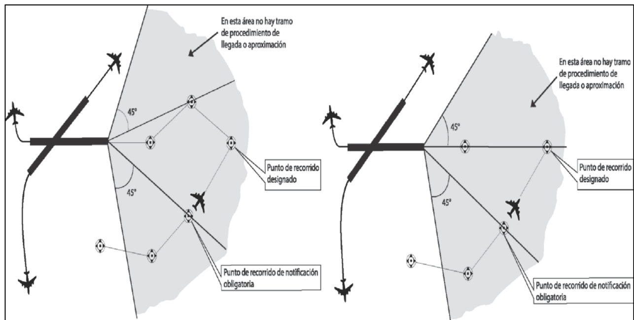
Figura 5-41. Área de protección de llegada
