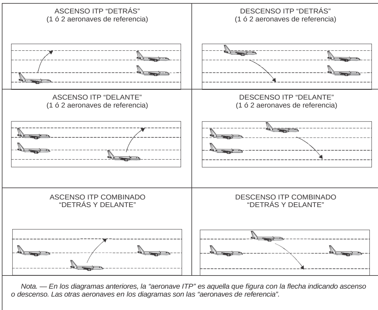
Figura 5-29. Escenarios de cambio de nivel de vuelo ITP (véase 5.4.2.7.3)
