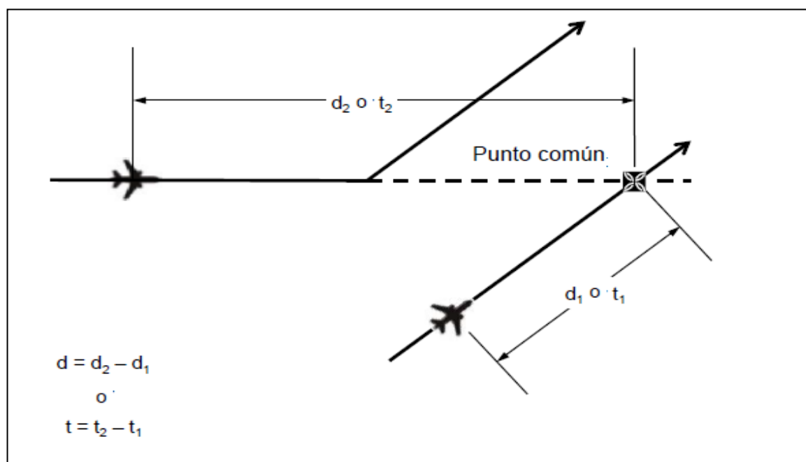
Figura 5-33. Cálculo de la distancia/tiempo longitudinal entre aeronaves — misma derrota prevista, pero no idéntica [véase 5.4.2.9.5 b)]
