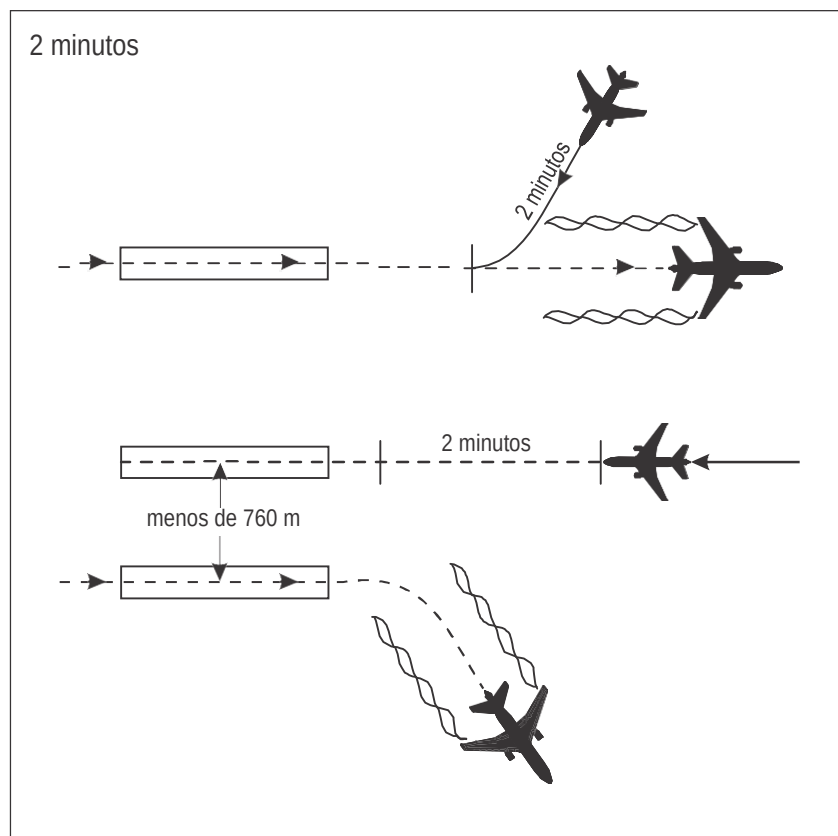
Figura 5-46. Separación de 2 minutos por estela turbulenta para aterrizajes en sentidos opuestos [véase 5.8.5 b)]
