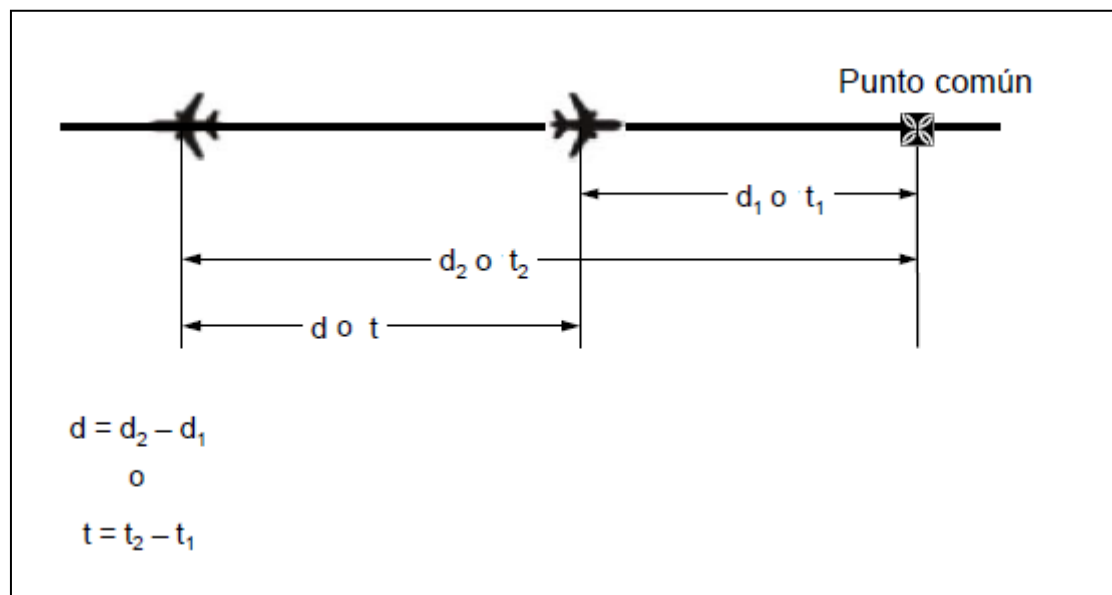
Figura 5-31. Cálculo de la distancia/tiempo longitudinal entre aeronaves — derrota idéntica, sentido opuesto [véase 5.4.2.9.5 a)]
