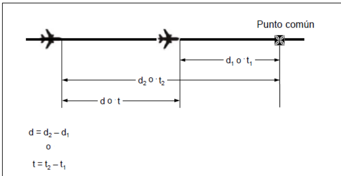
Figura 5-30. Cálculo de la distancia/tiempo longitudinal entre aeronaves — derrota idéntica, mismo sentido [véase 5.4.2.9.5 a)]
