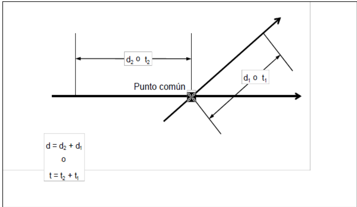
Figura 5-34. Cálculo de la distancia/tiempo longitudinal entre aeronaves — lados opuestos del punto común [véase 5.4.2.9.5 b)]
