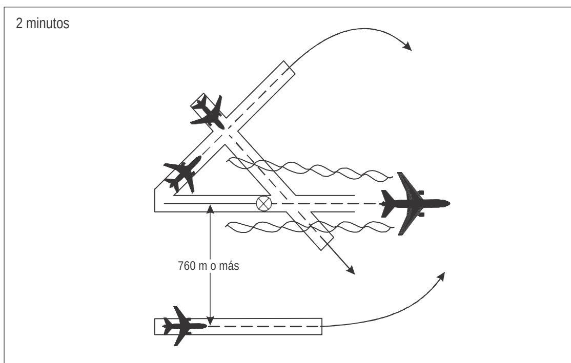
Figura 5-43. Separación de 2 minutos por estela turbulenta para aeronaves que se cruzan [véase 5.8.3.1 c) y d)]
